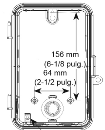
Terminal de tierra Caja Tipo 3R Figura 2
